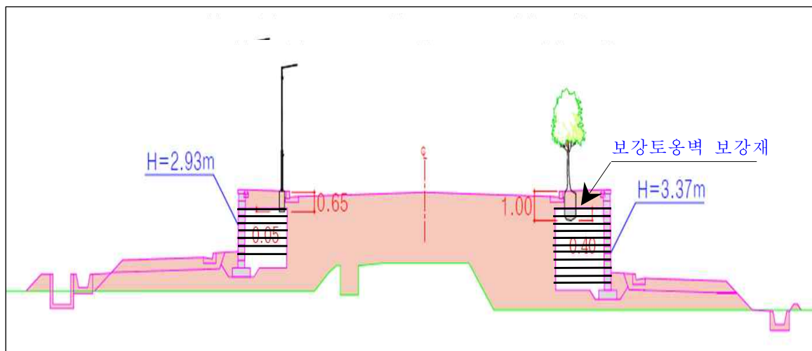
[그림1] 보강토옹벽 구간의 가로등 및 가로수 설치 계획
