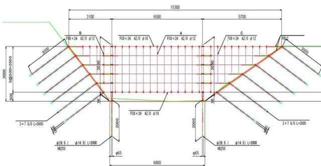
▲ 설계도면
